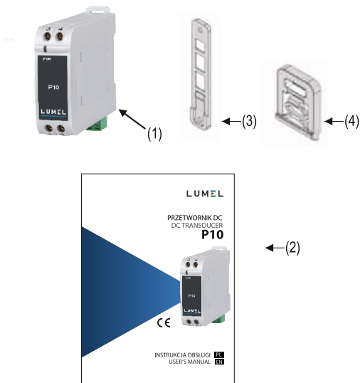
Rys. 1. Zestaw przetwornika.
